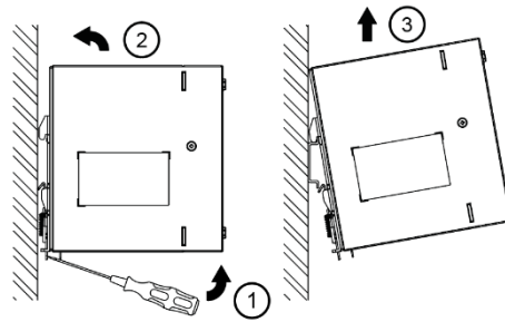
图. 3.2 拆卸
