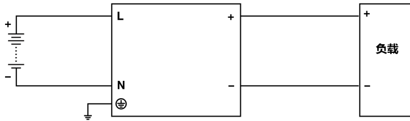
图. 4 DC 输入接线示意图
