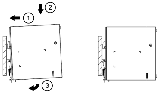
图. 3.1 安装
