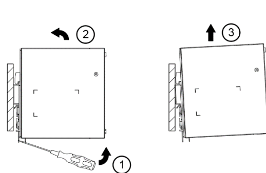
图. 3.2 拆卸
