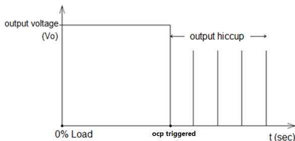
图 6. OLP/OCP 下进入打嗝模式
