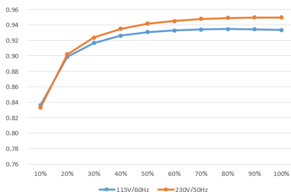
图 2. 24 V (max. 200 W) 机种典型效率曲线
