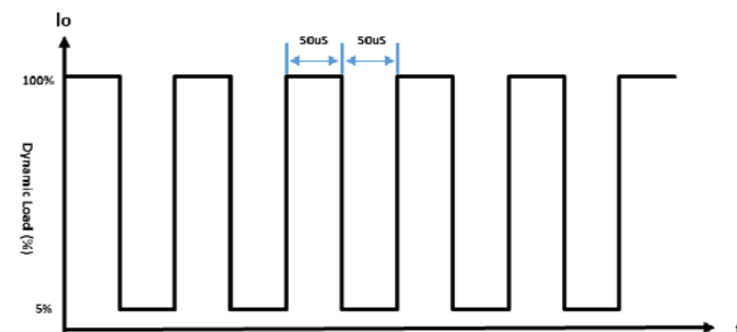
图 5-2. 动态负载
