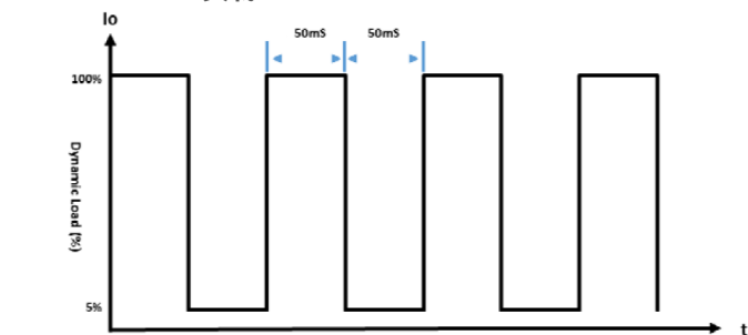
图 5-1. 动态负载
